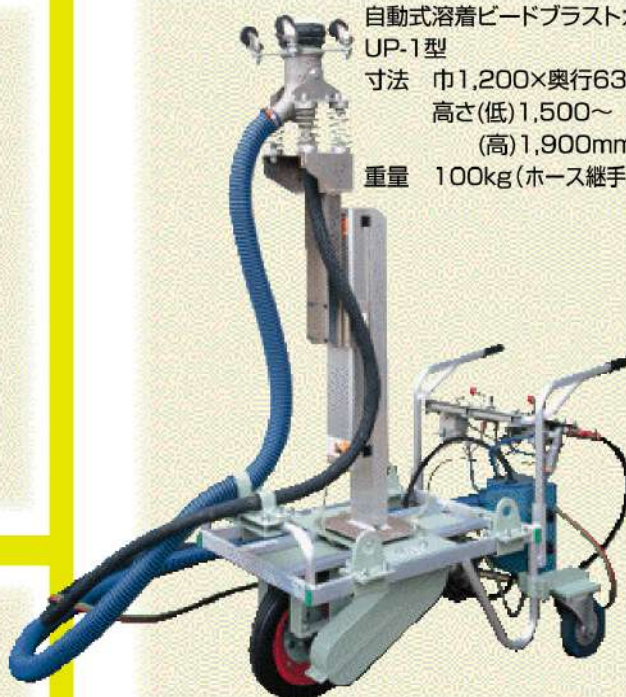
ロング専用ブラストガン LONJI-802型 寸法 巾800×奥行600×高さ270mm 重量 43kg
